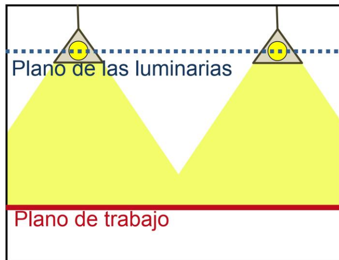
Ilustración 11 - Plano de Trabajo. Fuente: Castilla Cabanes, Nuria, Blanca Giménez, Vicente, Martínez Antón, Alicia, Pastor Villa, Rosa María – LUMINOTECNIA.
