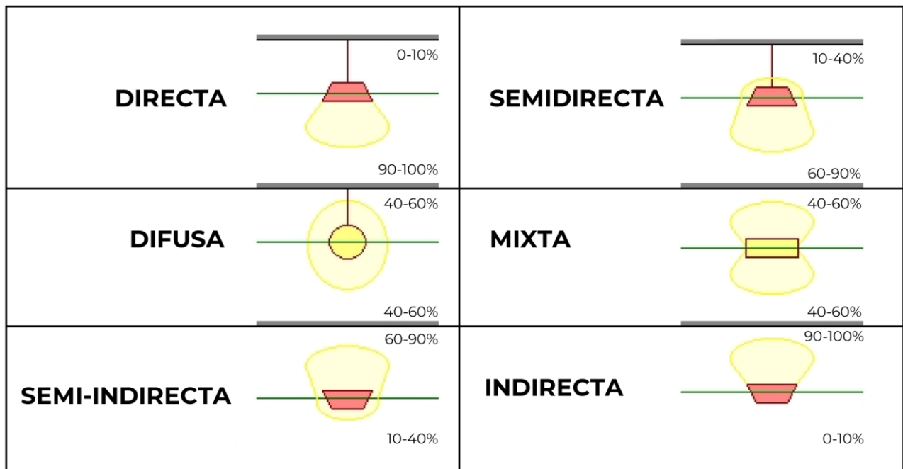
Ilustración 10 - Tipos de iluminación. Fuente: Docente Investigador tomando como base la clasificación de CIE según su distribución de luz.
