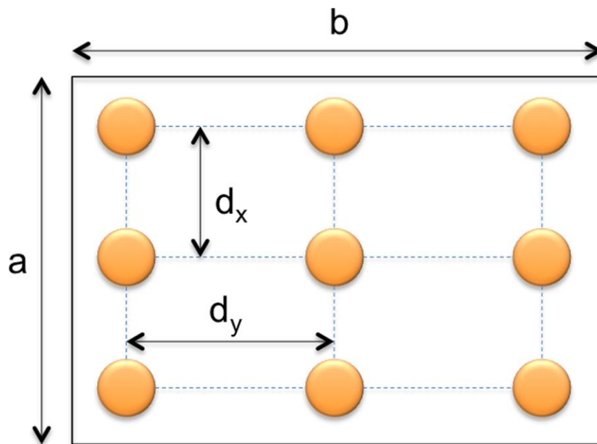
Ilustración 12 - Esquema de emplazamiento de luminarias. Fuente: https://grlum.dpe.upc.edu/manual/disenioProyecto-predimensionado.php
