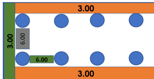
Ilustración 18 - Paso 8 - emplazamiento entre luminarias. Fuente: Docentes Investigadores.
