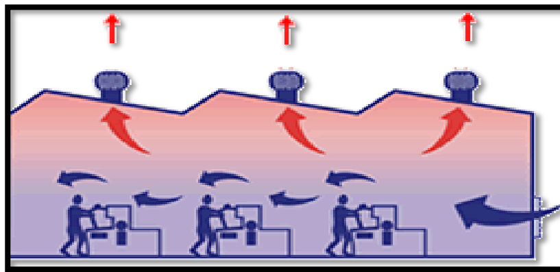
Figura. 34 Distribución del aire por medio de los extractores eólicos.
