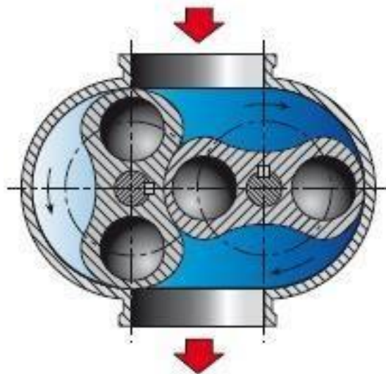
FIGURA 5. COMPRESOR TIPO ROOTS.
