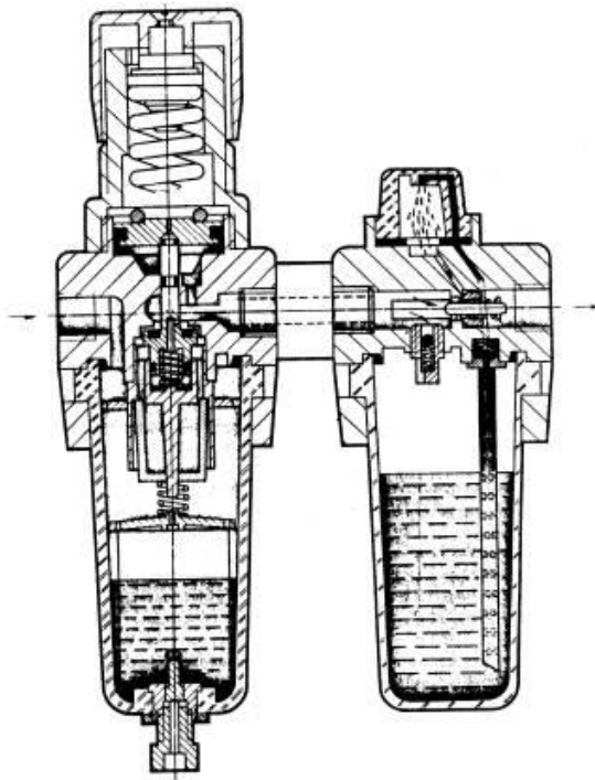
FIGURA 9. UNIDAD DE MANTENIMIENTO.
