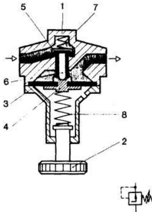
FIGURA 13. REGULADOR DE PRESIÓN SIN ORIFICIO DE ESCAPE
