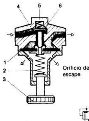
FIGURA 12. REGULADOR DE PRESIÓN CON ORIFICIO DE ESCAPE
