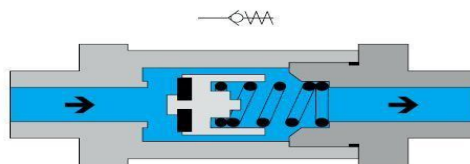
FIGURA 20. VÁLVULA ANTI RETORNO
