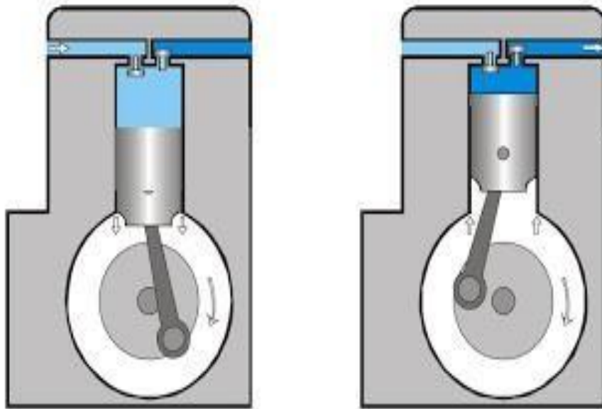
FIGURA 2. COMPRESOR DE ÉMBOLO O DE PISTÓN.
