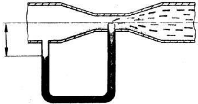
FIGURA 14. LUBRICADOR.
