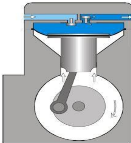
FIGURA 3. COMPRESOR DE MEMBRANA.
