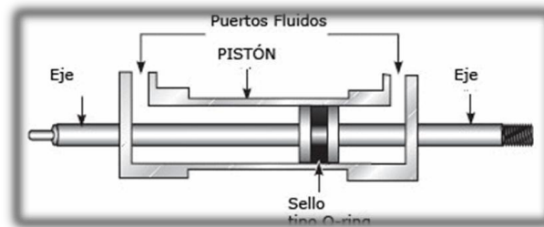
FIGURA 28. CILINDRO DE DOBLE VÁSTAGO.
