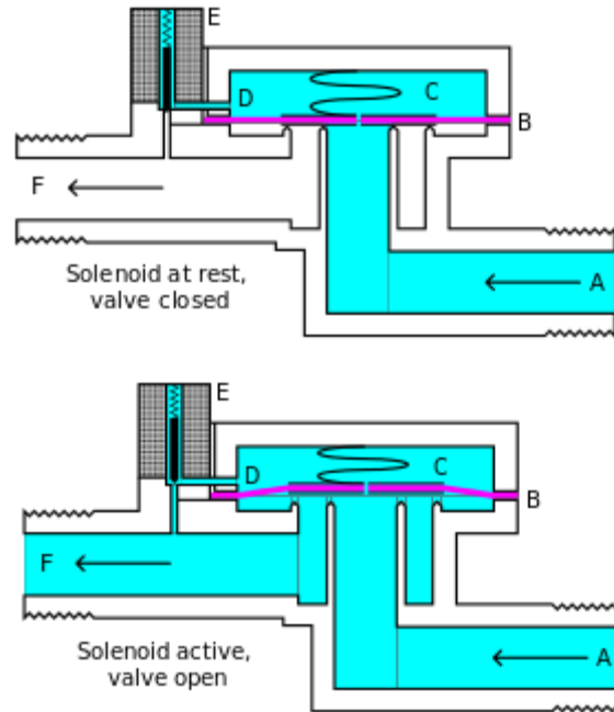
FIGURA 22. ELECTROVÁLVULAS.
