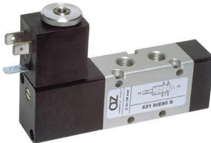
FIGURA 24. ELECTROVÁLVULAS DE CINCO VÍAS.
