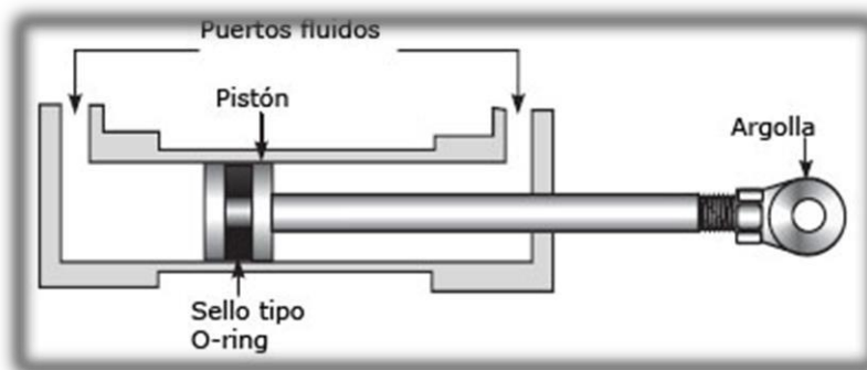
FIGURA 27. CILINDRO DOBLE EFECTO.
