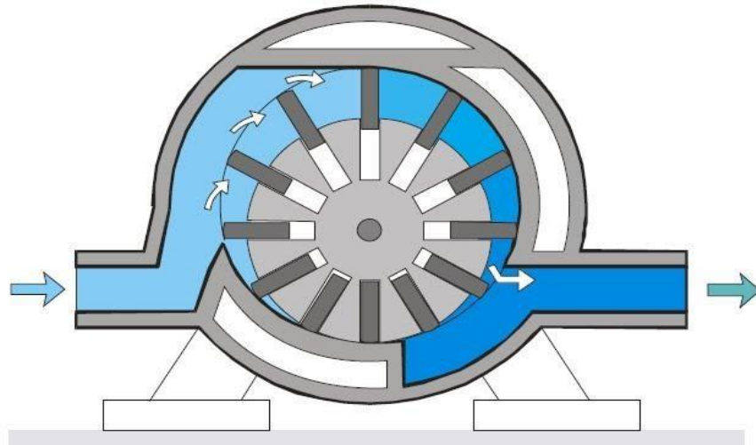
FIGURA 4. COMPRESOR DE PALETAS.
