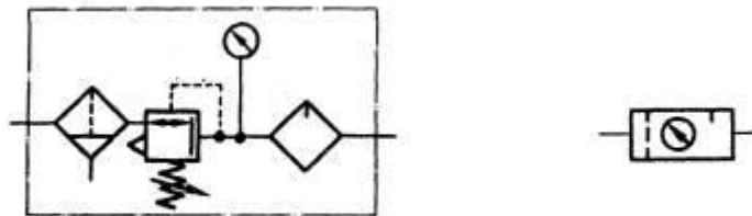
FIGURA 9. UNIDAD DE MANTENIMIENTO.
