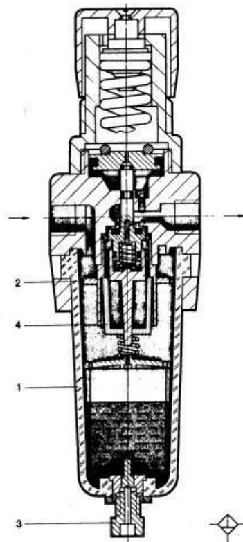
FIG. 11. CAMINO DEL AIRE A TRAVÉS DEL FILTRO.
