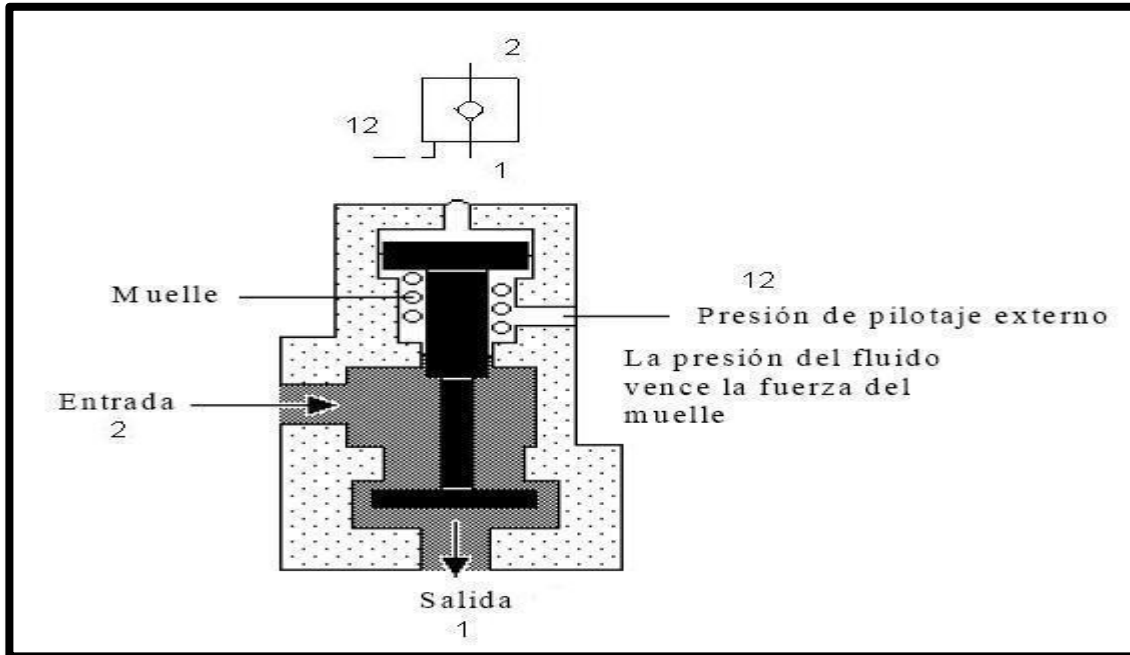
FIGURA 21. VÁLVULA ANTI RETORNO PILOTADA
