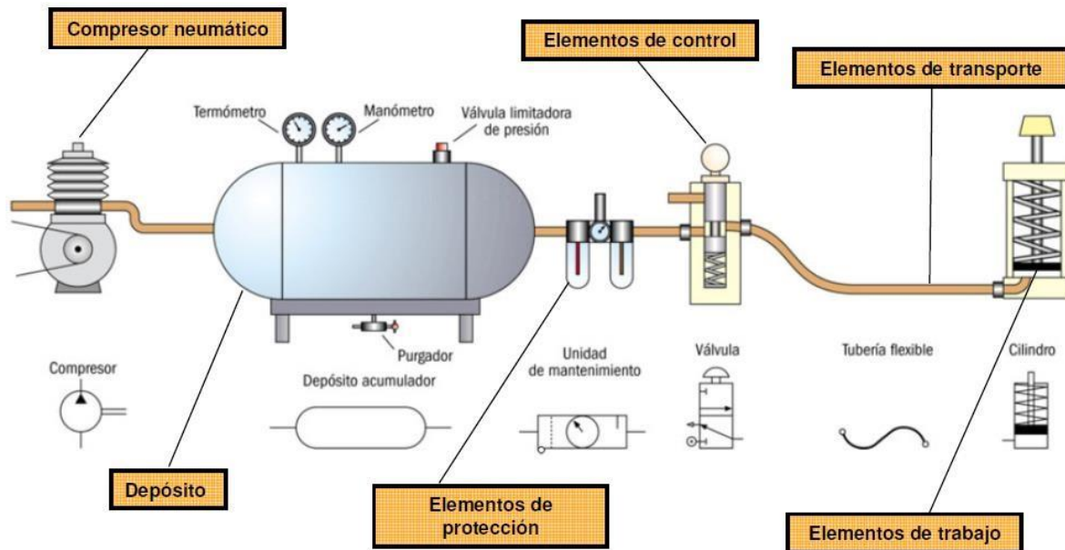
FIGURA 1. SISTEMA NEUMÁTICO
