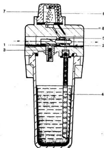
FIGURA 15. COMO EL AIRE COMPRIMIDO ATRAVIESA EL ACEITADOR.
