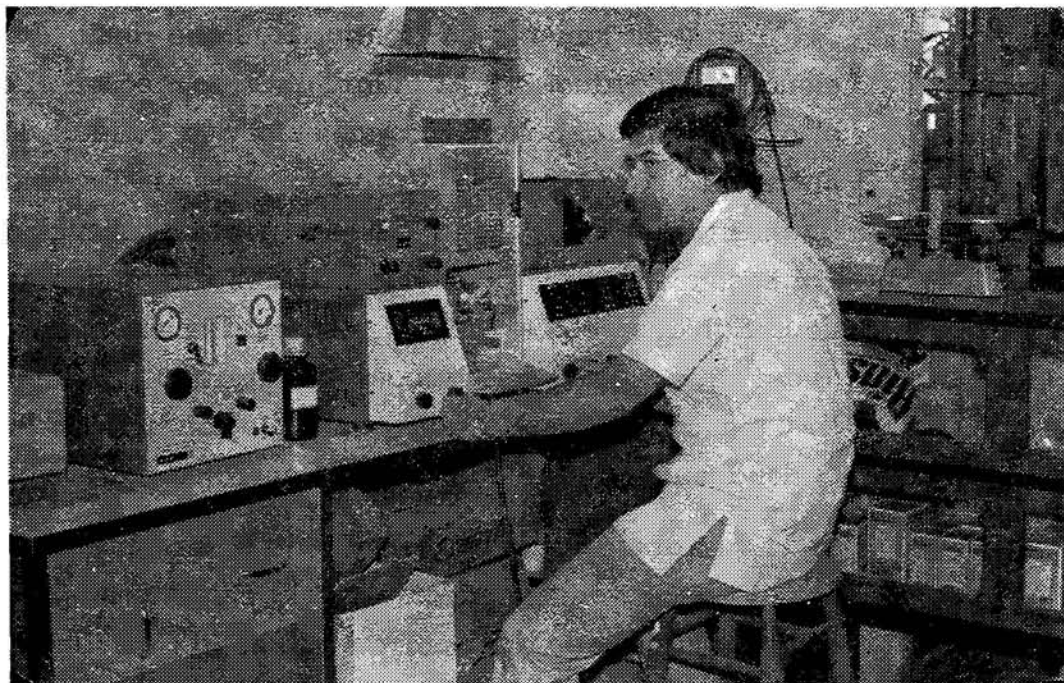
La fotografía muestra el ESPECTROFOTOMETRO DE ABSORCION ATOMICA que sirve para determinar, mediante las lámparas que utiliza, las concentraciones del elemento por analizar ya sea, presencia de hierro, manganeso, o fluoruros, en la muestra de Agua que se esta analizando. Opera el aparato el Lic. Francisco Mendoza, Químico Farmacéutico, (Jefe del Depto.)..
