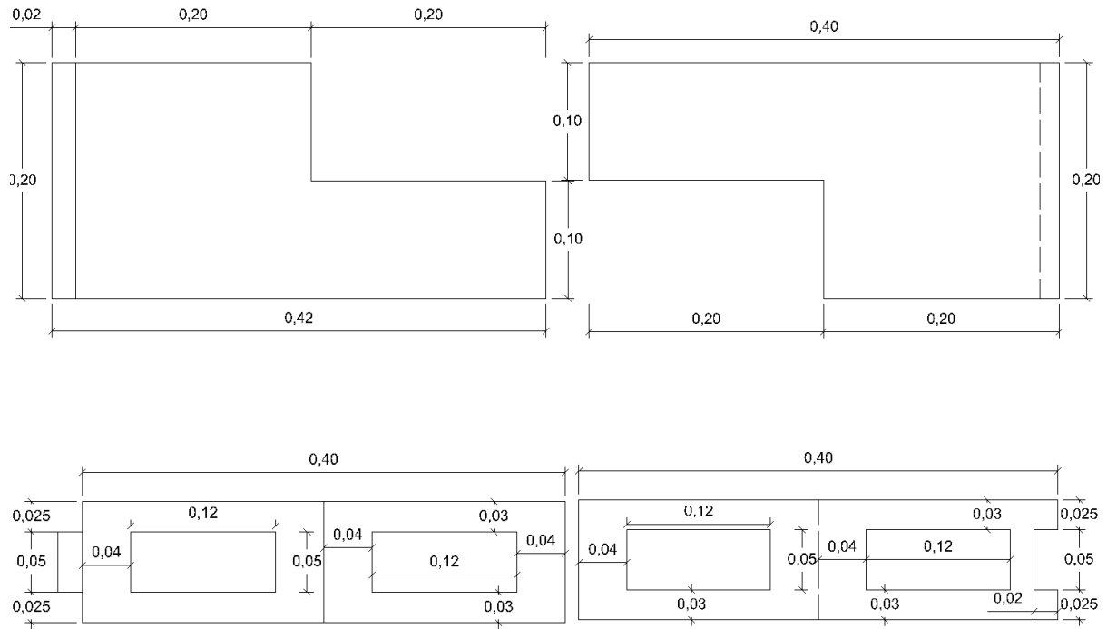
Figura 39. Vistas en 2D de propuesta de bloque de plástico. Fuente: diseño propio, 2018
