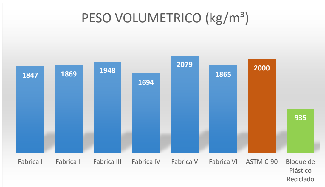
Grafica No.1. Comparativo de la densidad del bloque de concreto versus el de plástico. Fuente: elaboración propia, 2018
