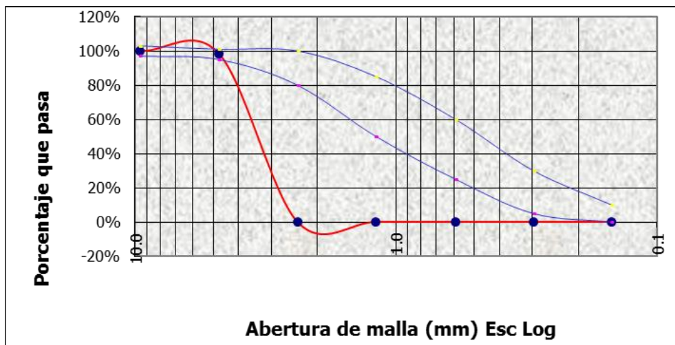
Figura 21. Resultado de granulometría realizada al plástico de polietileno peletizado.
