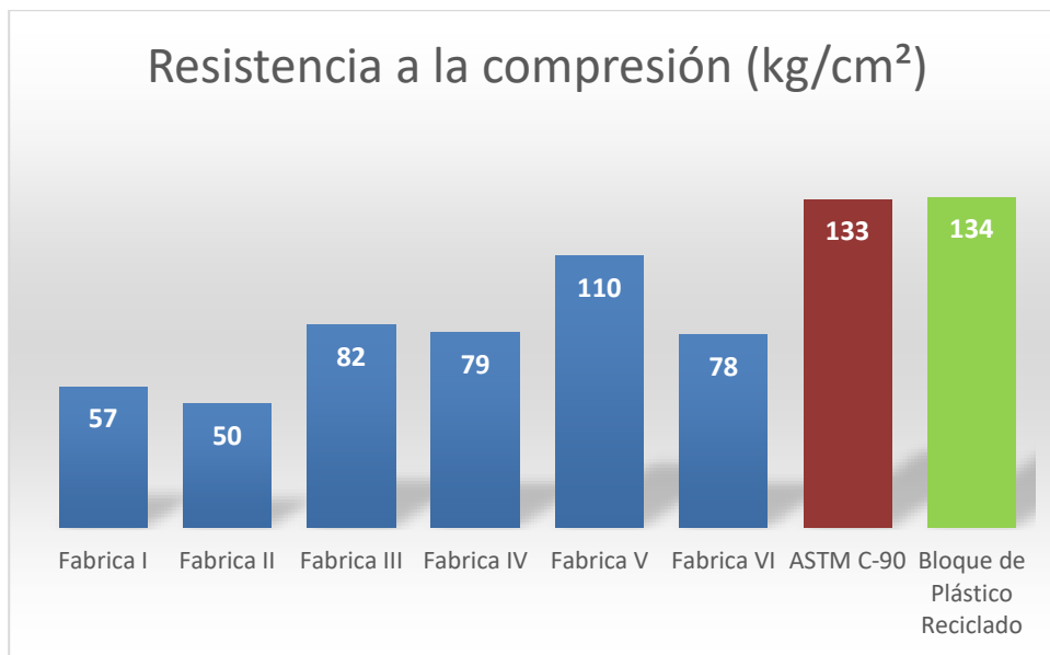
Grafico No.2. Comparativo de la resistencia a la compresión del bloque de concreto versus el de plástico. Fuente: elaboración propia, 2018
