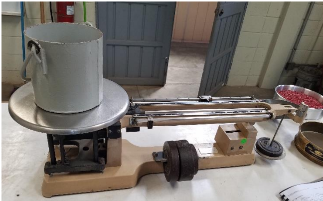
Figura 22. pesando molde a utilizar para prueba
