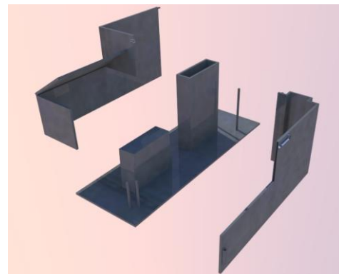
Figura 41. Se muestra las 3 partes desensambladas del molde.
