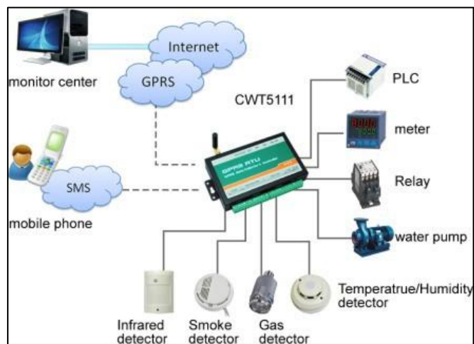
Figura 18: Sistema de monitoreo en tiempo real
