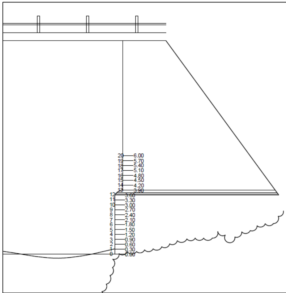
Figura 11: Escala de medición en un extremo del puente Urbina
