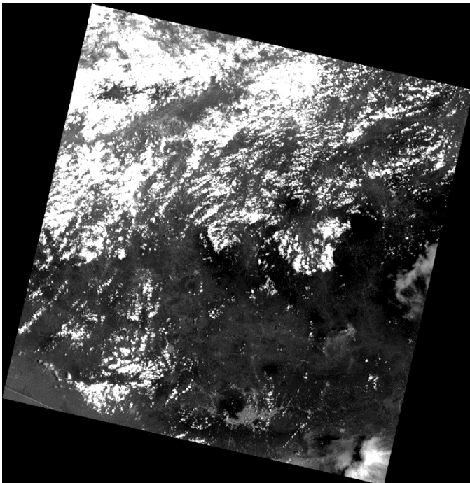
Figura 21. Imagen Landsat 8, cuadrante 019050 correspondiente al mes de agosto de 2015. Fuente: USGS (s.f.). EarthExplorer – Home. Recuperado de: https://earthexplorer.usgs.gov/
