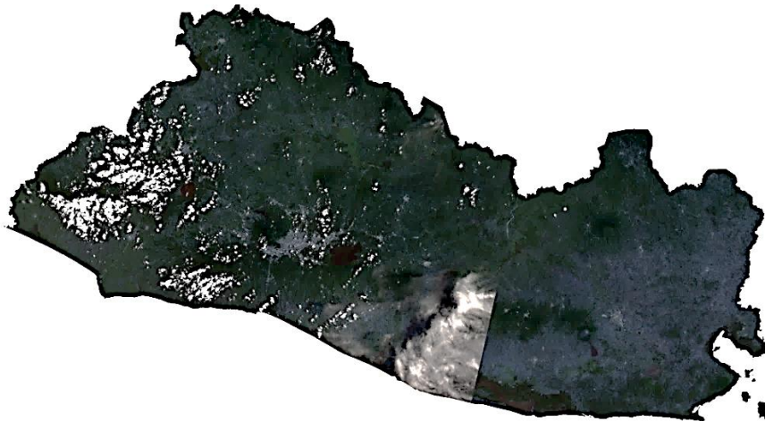
Figura 25. Imagen Landsat 8, con cuadrantes unidos y recortada correspondiente al mes de agosto de 2015.
